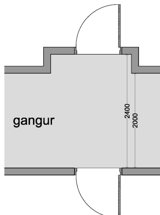
Mynd 2. Gangur breidd 2,0 m. Öll mál í mm
