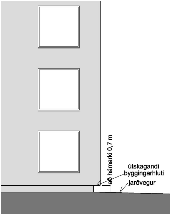
Mynd 3. Dæmi um útskagandi byggingarluta minna en 0,7 m frá jörðu
