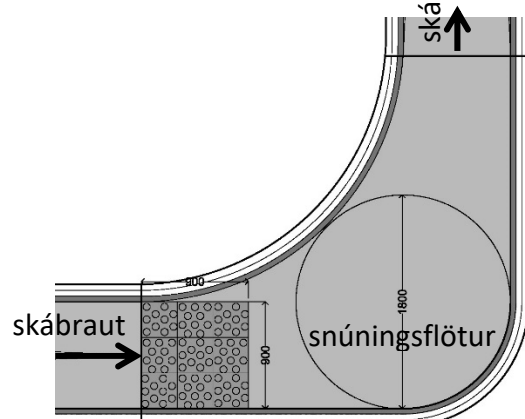
Mynd 5. Dæmi um snúningsflöt, öll mál í mm
