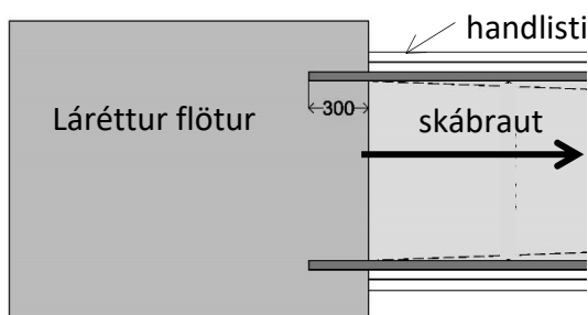
Mynd 11. Dæmi um handlista sem fer 300 mm fram fyrir skábraut
