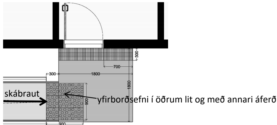
Mynd 13. Dæmi um hæðarmismun við skábraut, öll mál í mm
