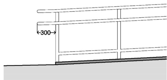
Mynd 12. Dæmi um snið í skábraut með handlista sem fer 300 mm fram fyrir enda skábrautar
