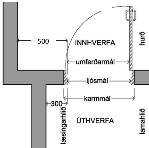
Mynd 1. Dæmi um hurð á lömum
