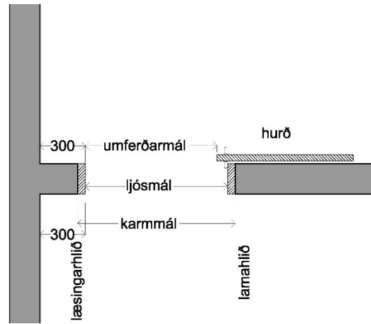
Mynd 2. Dæmi um rennihurð
