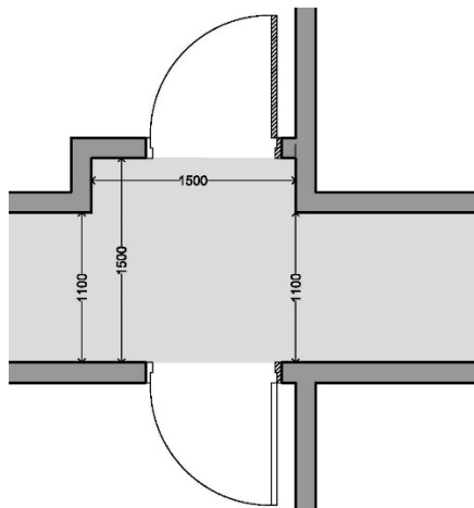
Mynd 3. Dæmi um gang með 1,50 m x 1,50 m útskoti, öll mál í mm
