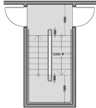
Mynd 3. Stigabreidd 1,00 m í íbúðarhúsnaði með lyftu fyrir sjúkrabörur. Öll mál í mm
