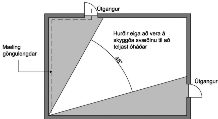
Mynd 2. Útskýring á óháðum flóttaleiðum.
