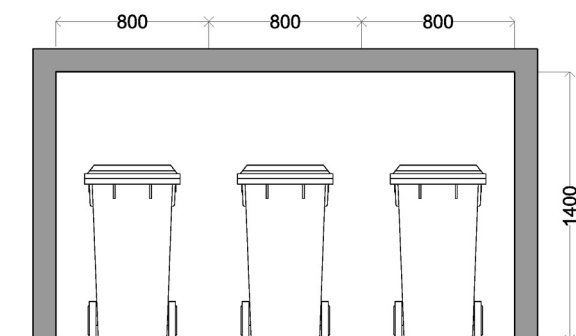
Mynd 1. Sorpgeymslur, öll mál í mm
