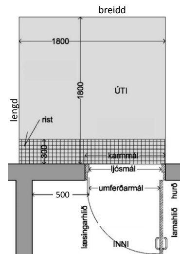
Mynd 4. Dæmi um pall/flöt með hurð sem opnast inn
