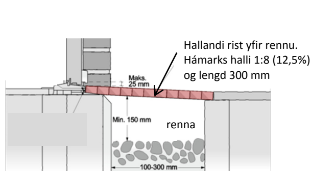
Mynd 11. Dæmi um rennu og rist við garðdyr
