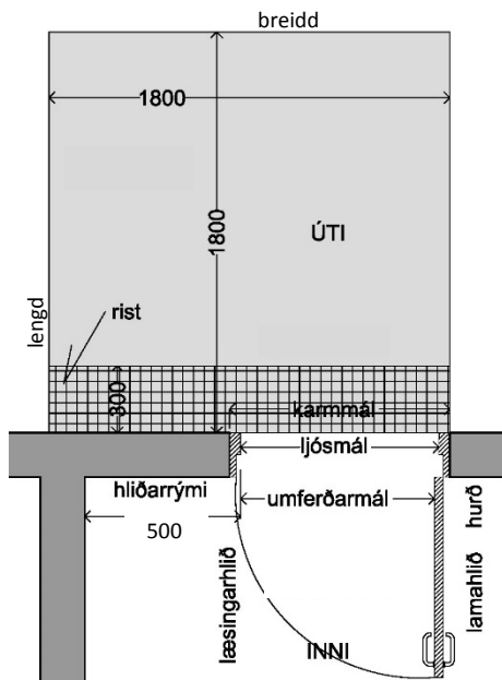
Mynd 10. Dæmi um hliðarrými við inngangshurðir
