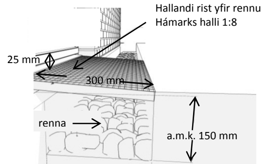
Mynd 12. Dæmi um rennu og rist við garðdyr
