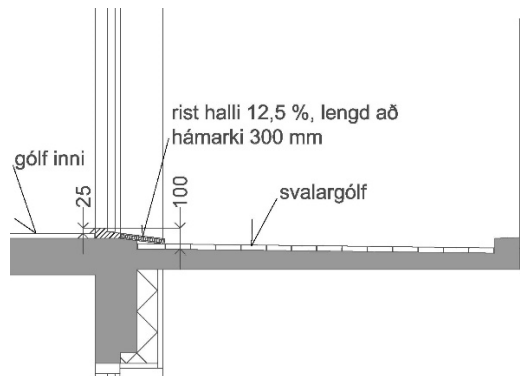
Mynd 12. Dæmi um frágang við svalardyr, sneiðing
