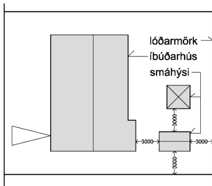
Mynd 1. Dæmi um staðsetningu smáhýsa á lóð. Öll mál í mm og eru þau lágmarksmál.
